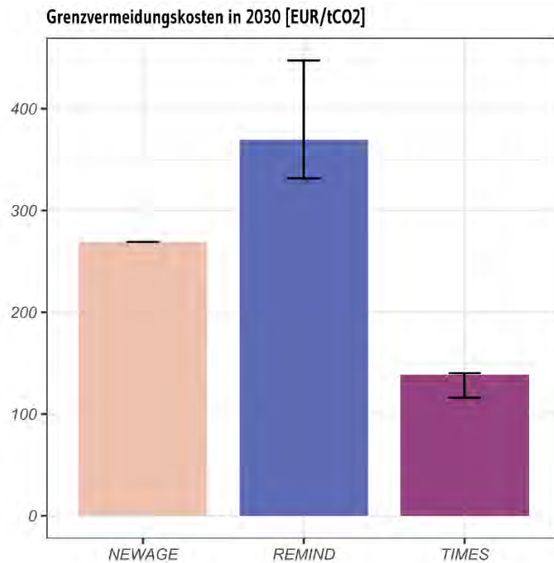
Abbildung 1.15: CO 2 -Grenzvermeidungskosten in 2030 für das Technologiemit-Szenario (Balken) und die anderen Zielerreichungsszenarien (Bandbreiten).
