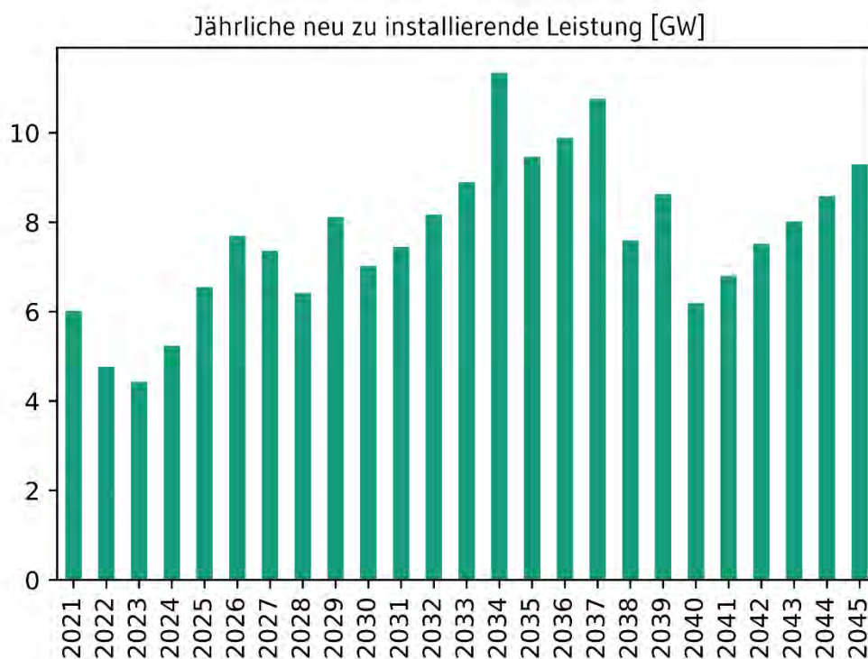
Abbildung 5.3: Neu zu installierende Leistung pro Jahr bis 2045 für das Fokus Wind-Szenario.
